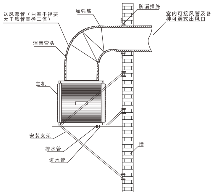
上出风机型挂墙安装图
